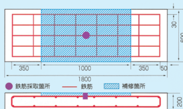
大型供試体配筋図 (補修前塩化物イオン量 4\text{kg/m}^3 )
